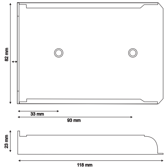
GP941 Halterung
